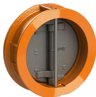
Valvole di ritegno doppio battente fino a 24"
